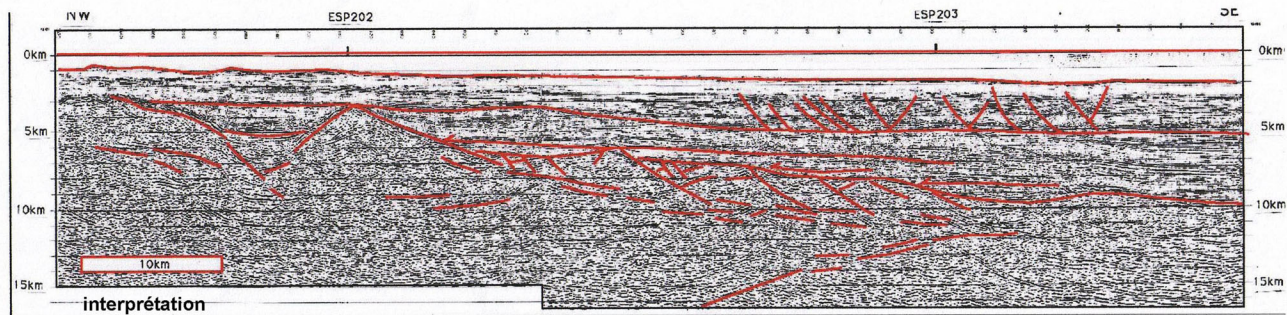
profil ECORS-1995-M.Seranne
