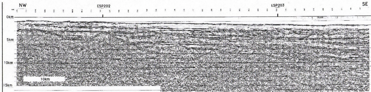
profil ECORS-1995-M.Seranne
